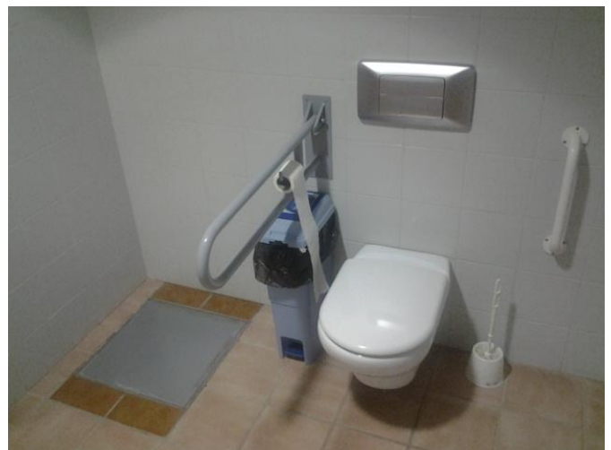
Cabina de aseo para PMR.
